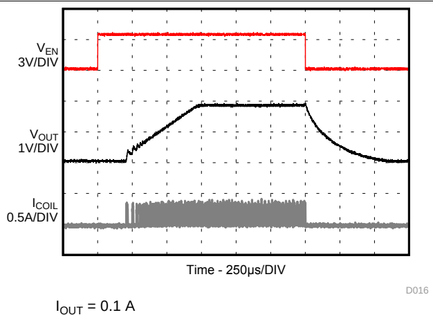
图 17. Startup with Load
