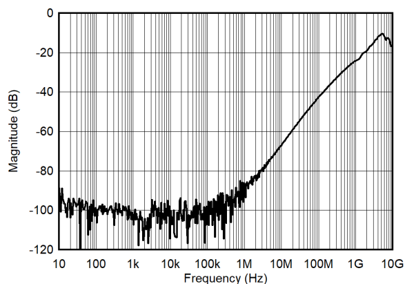
图 6-16. Off Isolation
