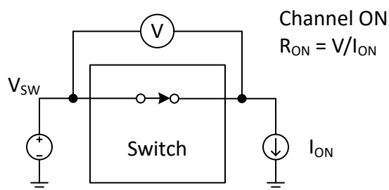
图 7-1. On Resistance
