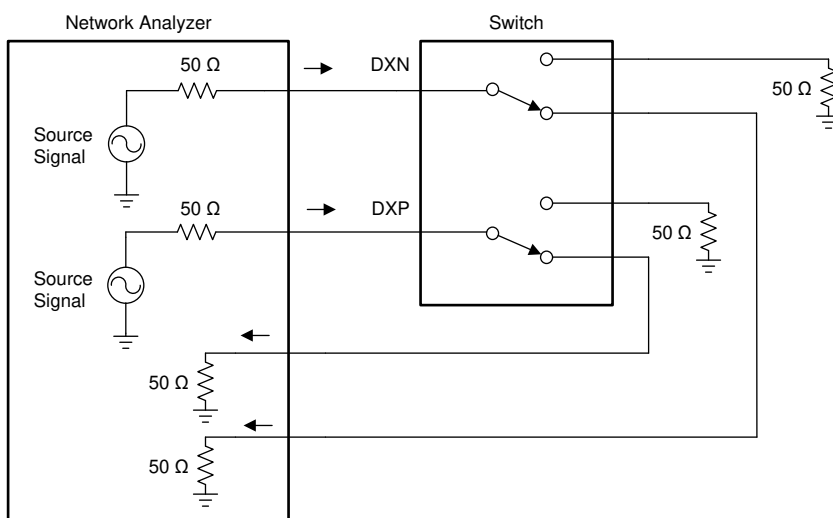
图 7-7. Crosstalk
