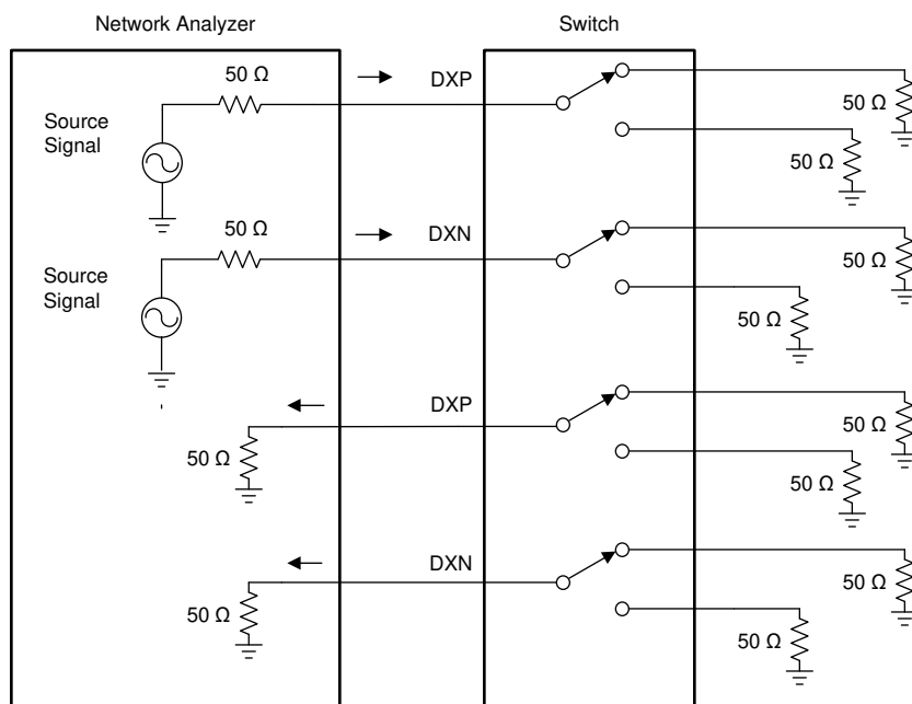
图 7-7. Crosstalk
