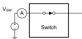
图 7-3. On Leakage
