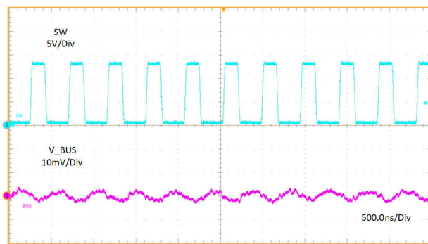
图 11-15. No Load Output Ripple
