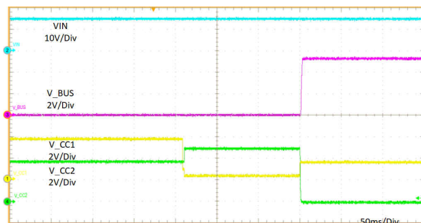
图 11-20. Rd Assert
