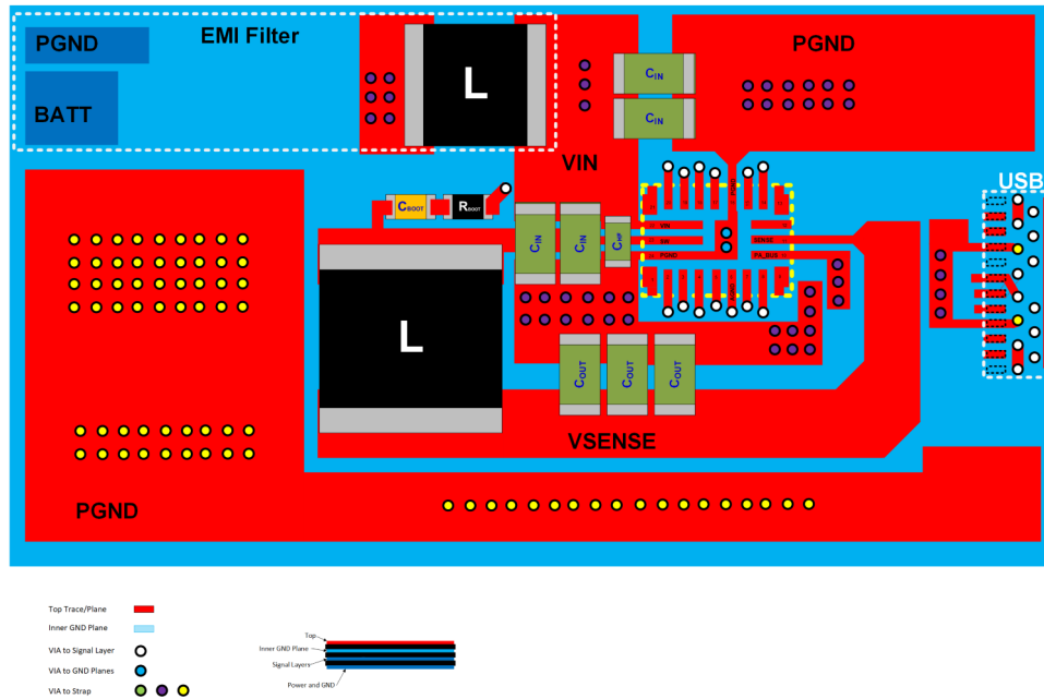
图 13-1. Layout Example
