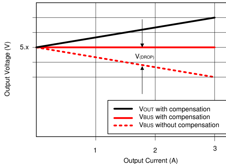
图 10-8. Voltage Drop
