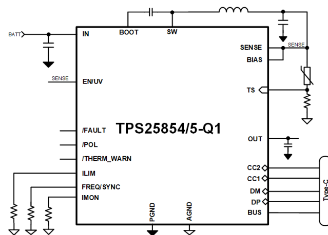
简化版原理图：TPS25854-Q1 和 TPS25855-Q1
