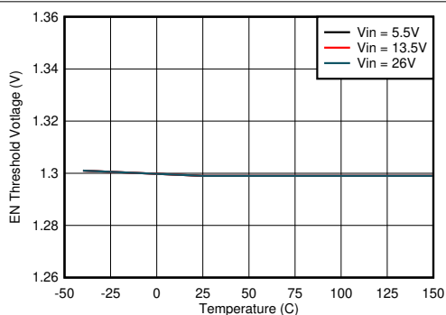
图 8-3. Precision Device Enable Threshold
