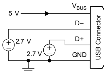
图 10-16. Divider 3 Mode
