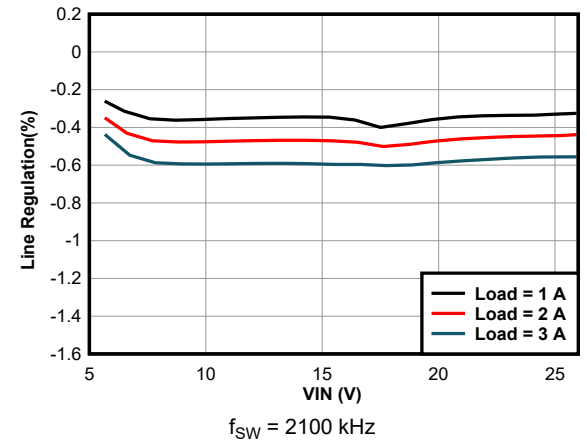
图 11-7. Line Regulation
