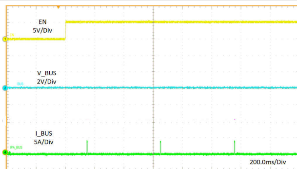
图 11-20. Rd Assert
