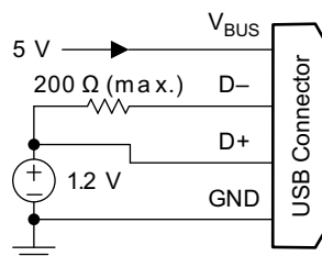
图 10-17. 1.2-V Mode
