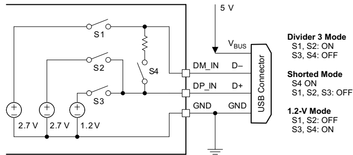
图 10-18. DCP Auto Mode
