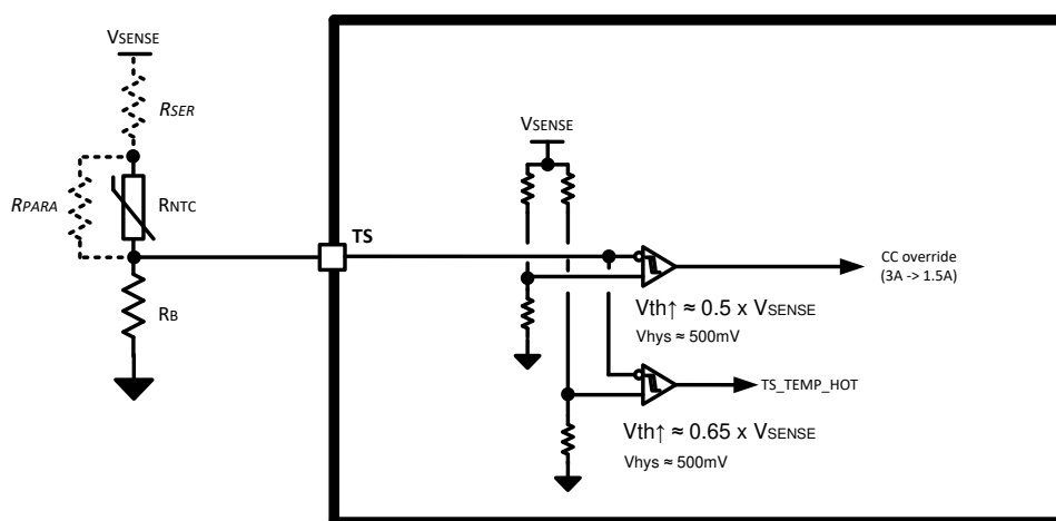
图 10-10. TS Input
