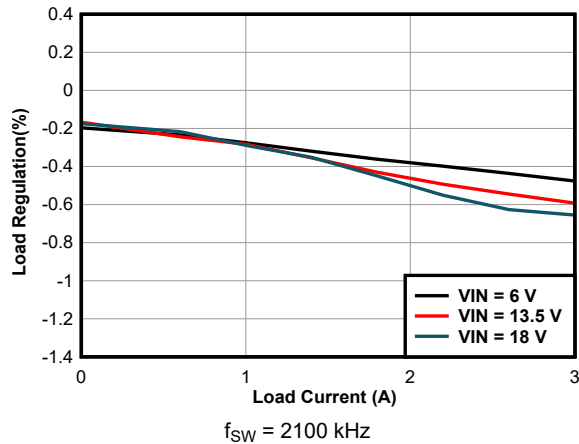
图 11-6. Load Regulation
