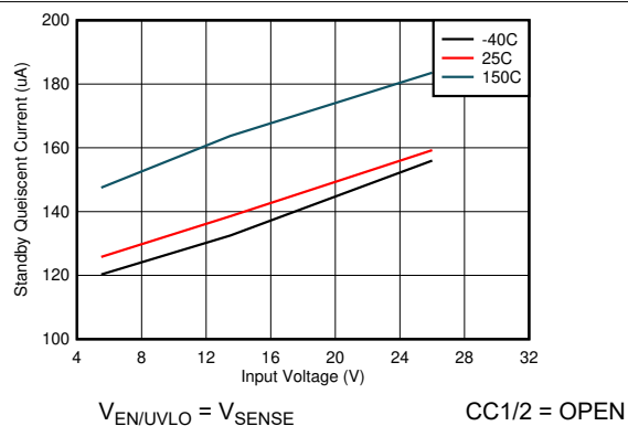
图 8-2. Standby Quiescent Current
