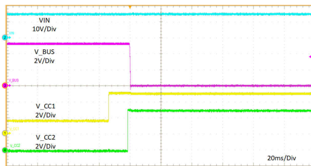
图 11-21. Rd Desert
