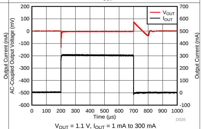
图 12. I_{OUT} Transient
