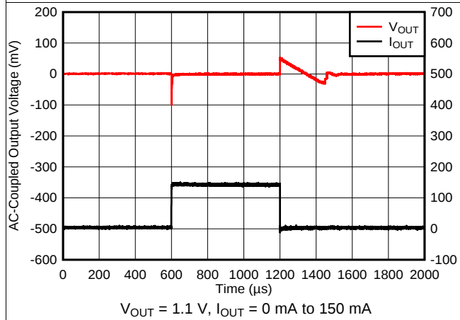
图 9. I_{OUT} Transient
