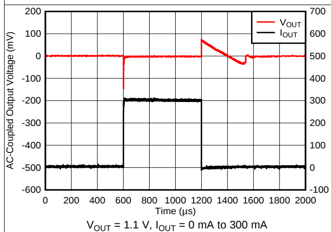
图 11. I_{OUT} Transient
