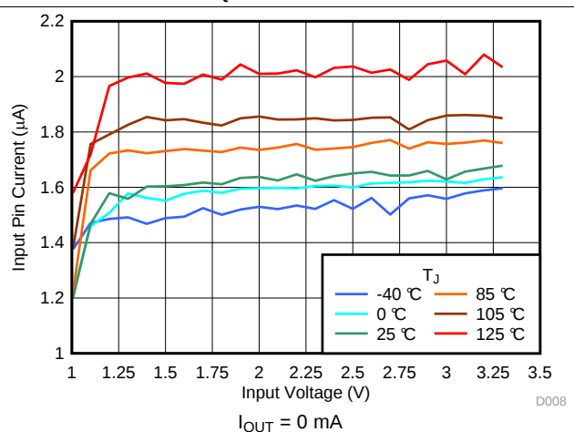
图 18. I_Q ( V_{IN} ) Over Temperature
