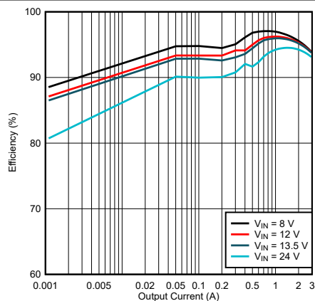
图 9-6. LM61430-Q1 Efficiency
