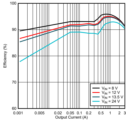
图 9-4. LM61430-Q1 Efficiency
