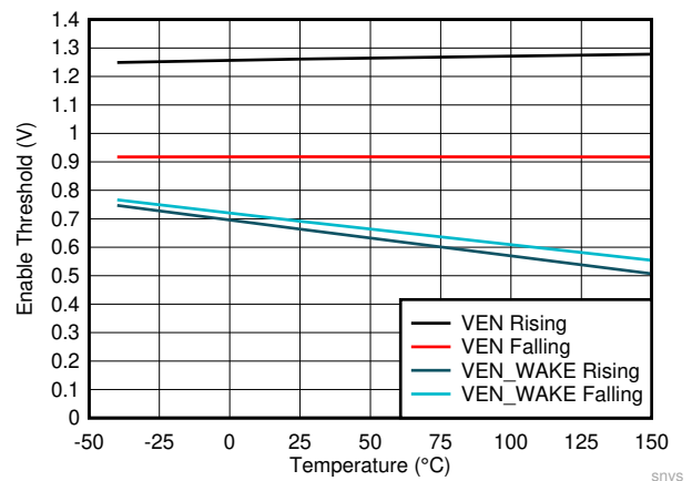
图 7-6. Enable Thresholds
