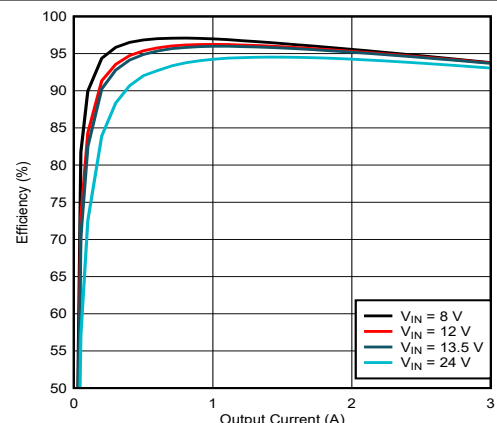
图 9-7. LM61430-Q1 Efficiency
