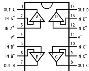
DGK 封装 14 引脚 TSSOP LMV934-N-Q1 顶视图
