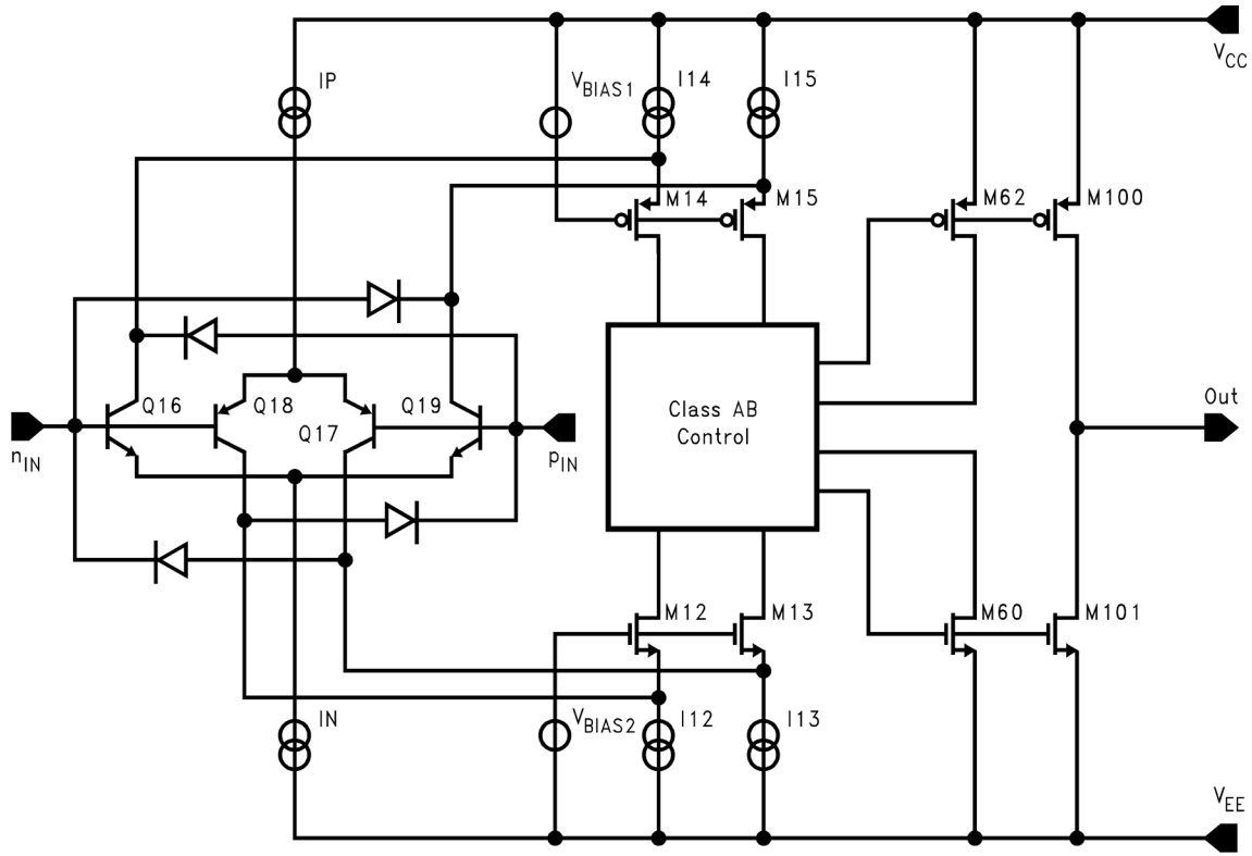
Figure 29. 简化原理图
