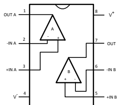
D 封装 8 引脚 SOIC LMV932-N-Q1 顶视图
