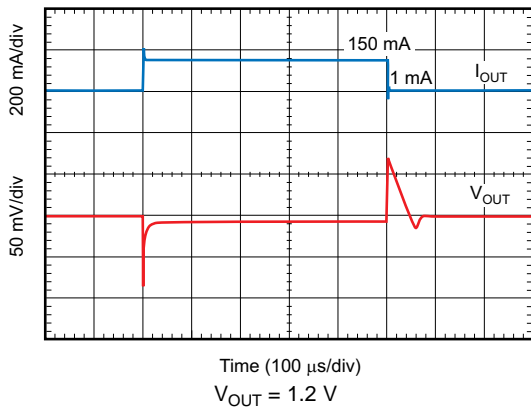
图 47. Load Transient Response
