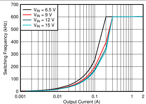
图 6-12. 开关频率与输出电流的关系, V OUT = 3.3V, L = 4.7µH
