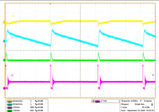
图 8-7. 稳态波形, I_{OUT} = 0.02A
