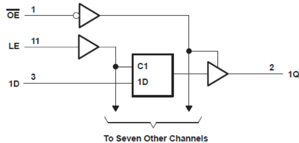
功能方框图
