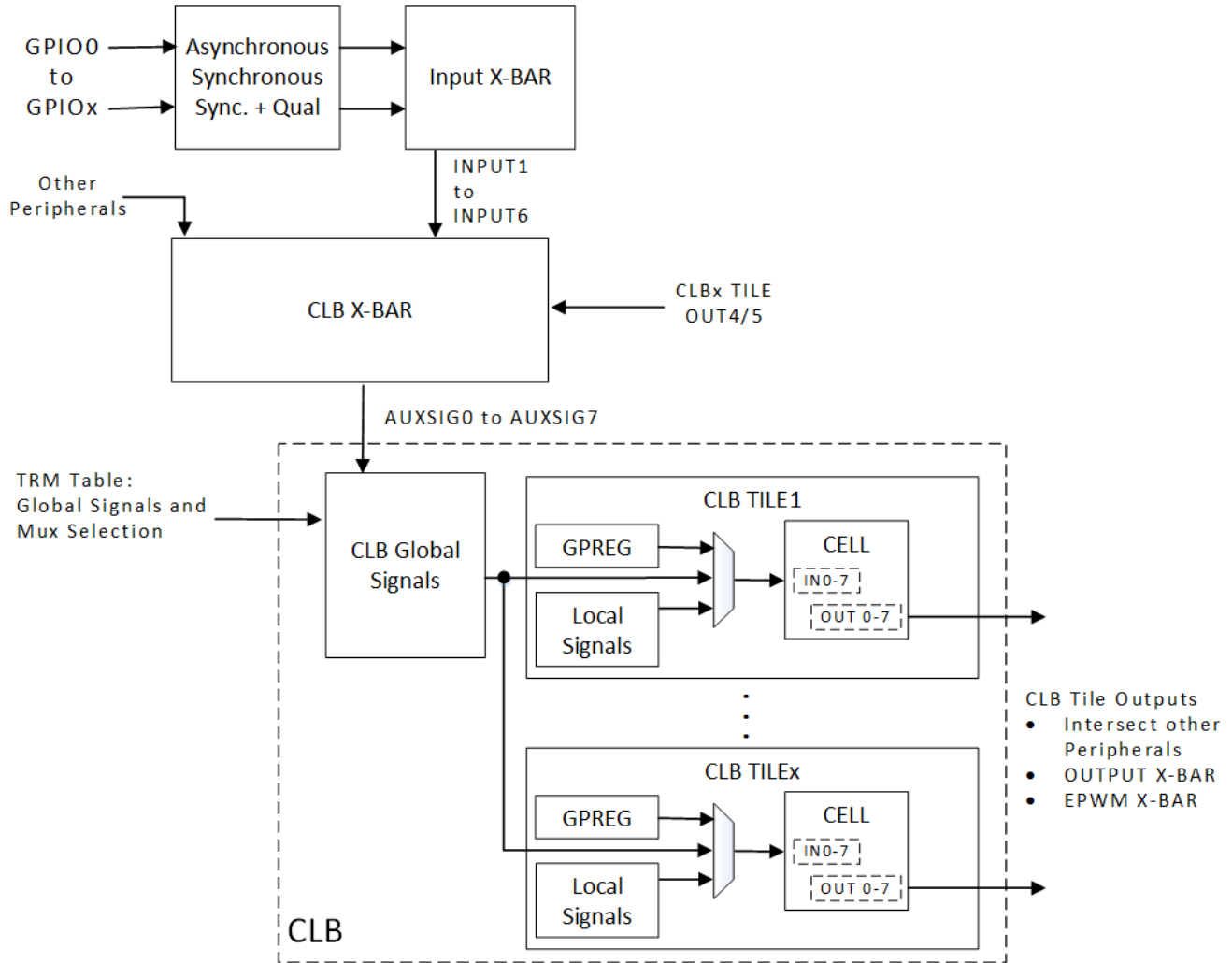
图 8-5. CLB Overview
