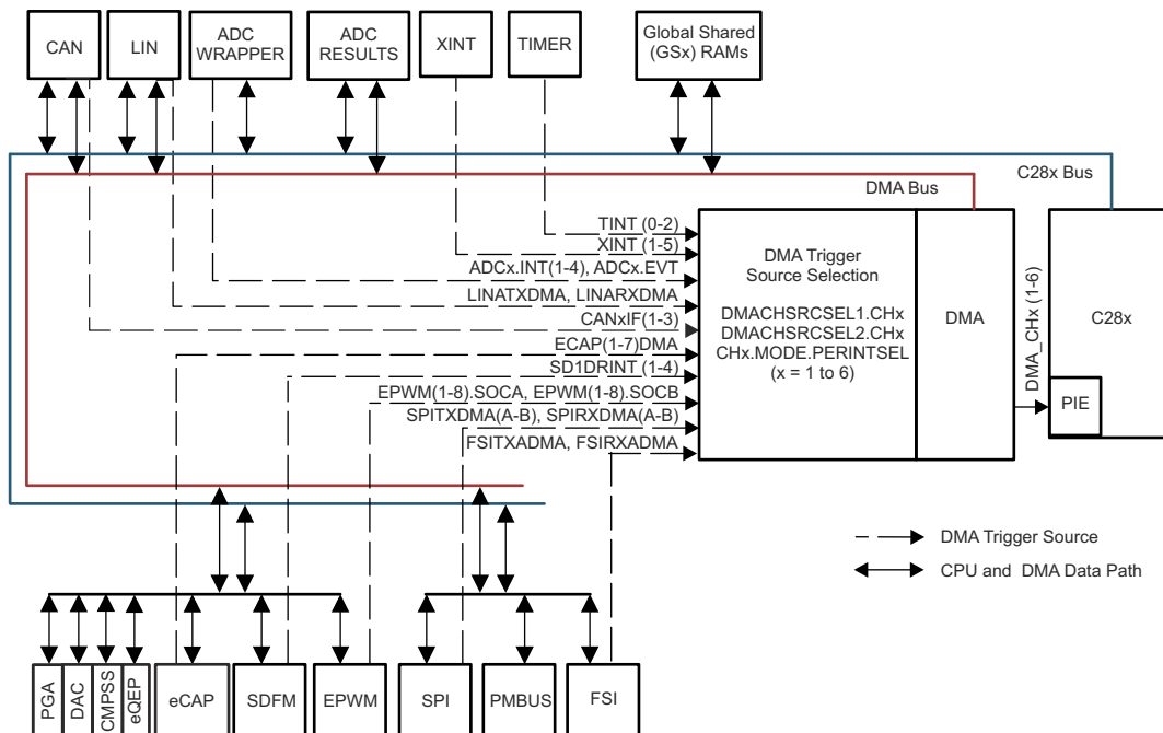
图 8-3. DMA Block Diagram
