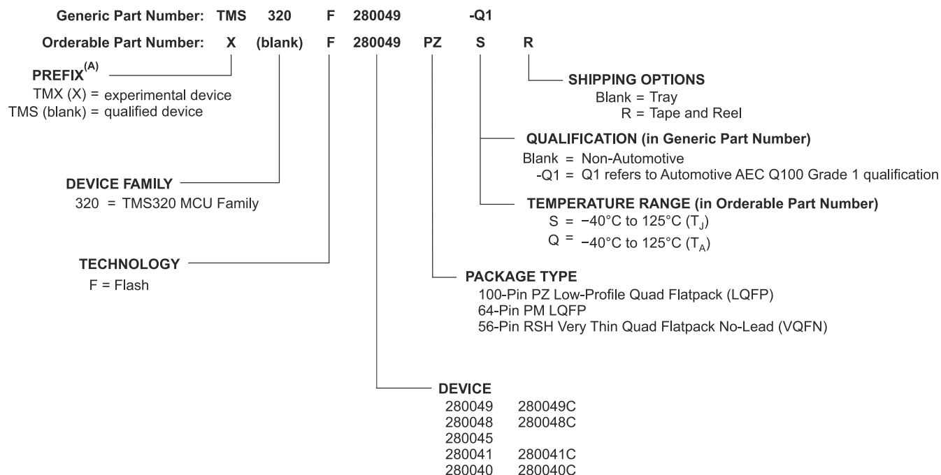
图 10-1. Device Nomenclature
