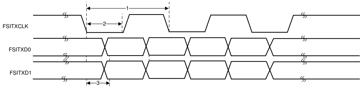
图 7-86. FSITX Timings
