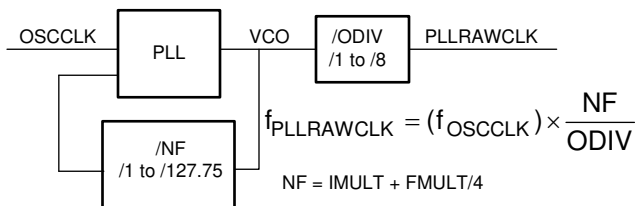
图 7-11. System PLL
