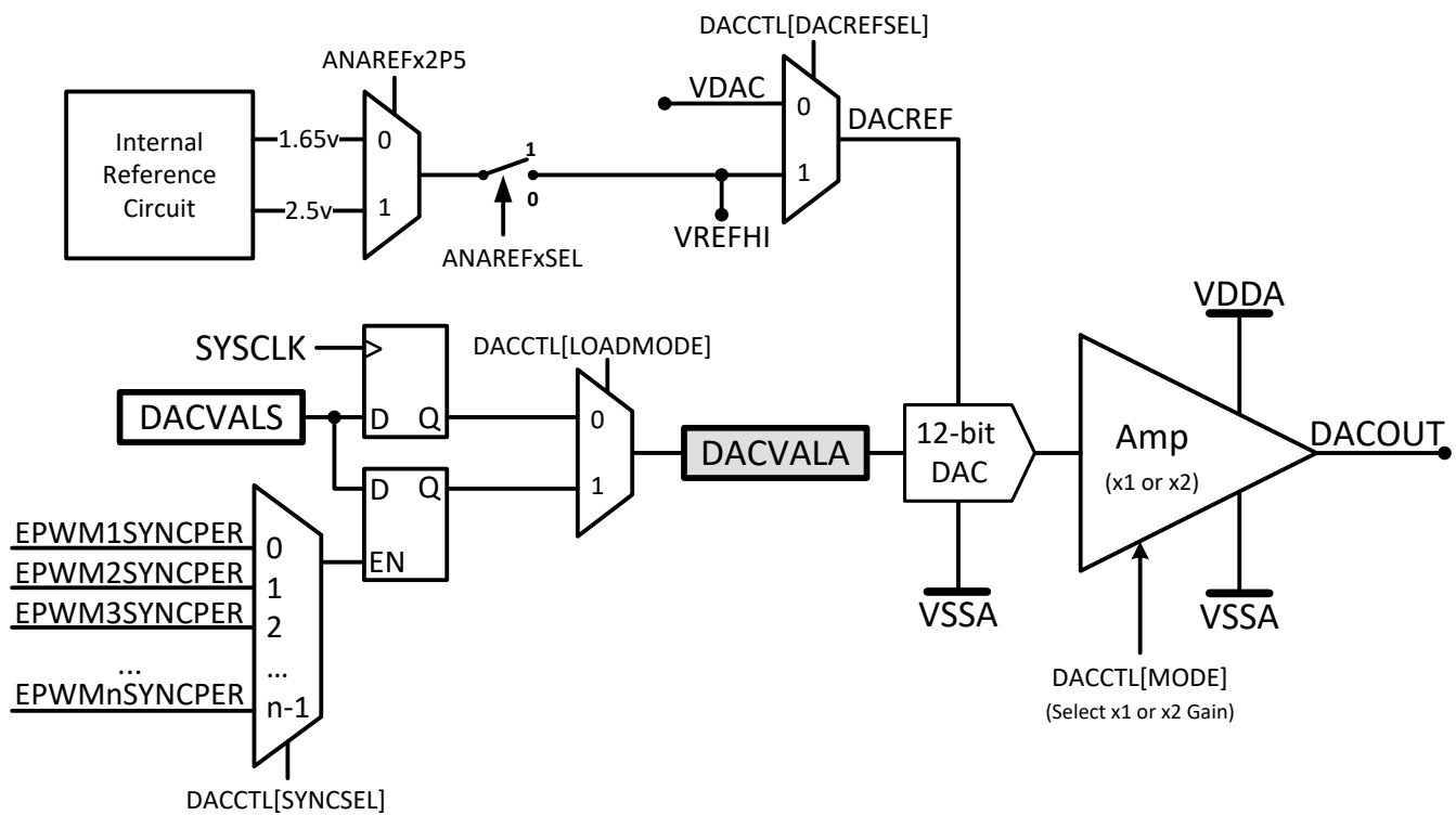
图 7-38. DAC Module Block Diagram
