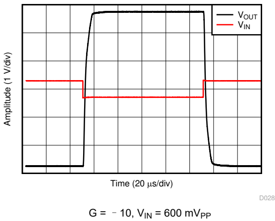
图 6-23. Overload Recovery
