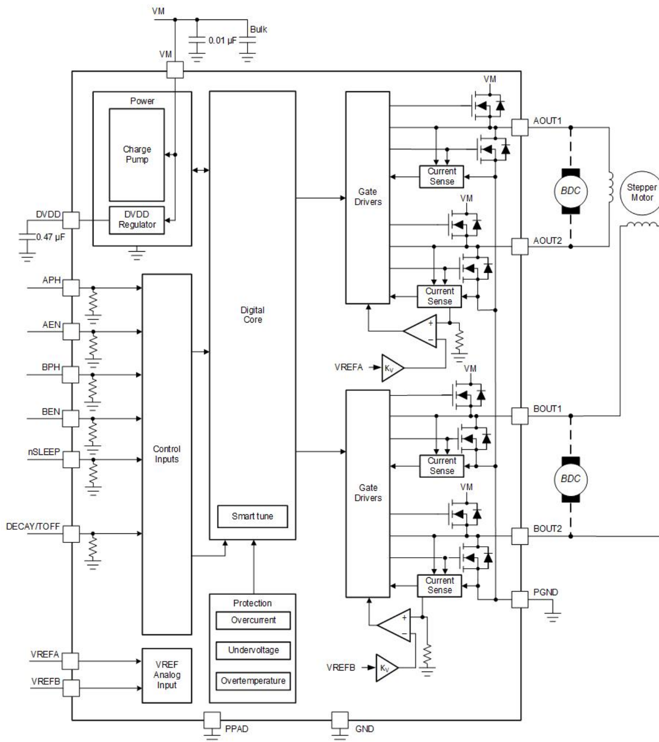
图 7-1. DRV8428E 方框图
