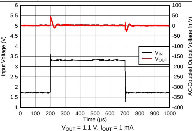
图 14. V_{IN} Transient
