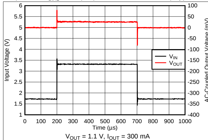
图 13. V_{IN} Transient
