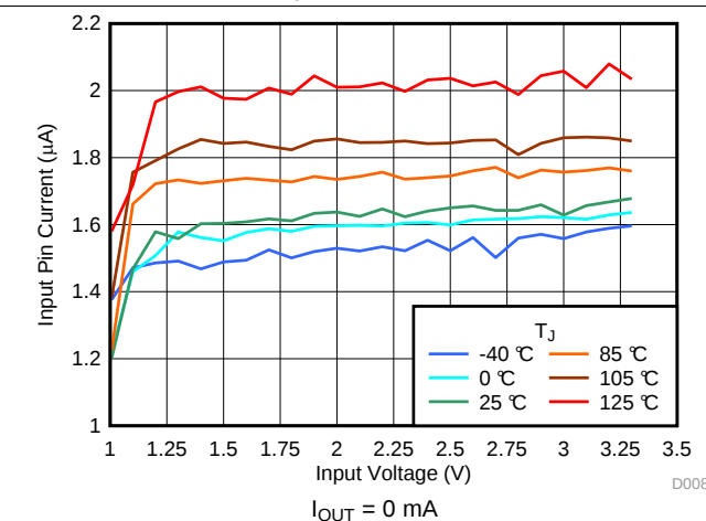
图 18. I_Q ( V_{IN} ) Over Temperature
