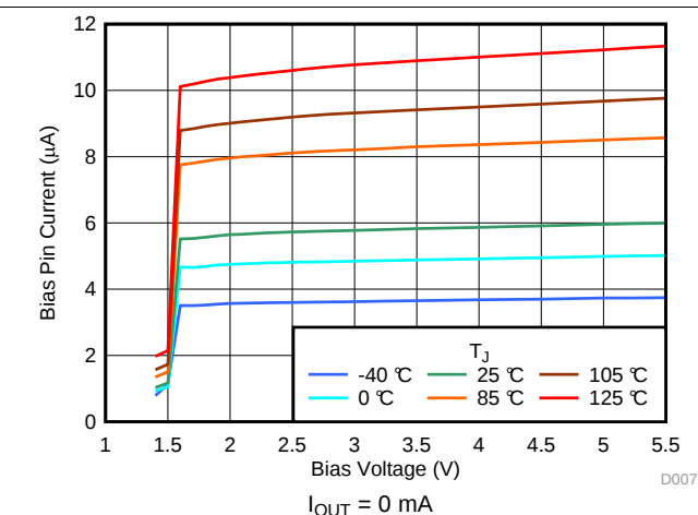
图 16. I_Q ( V_{BIAS} ) Over Temperature
