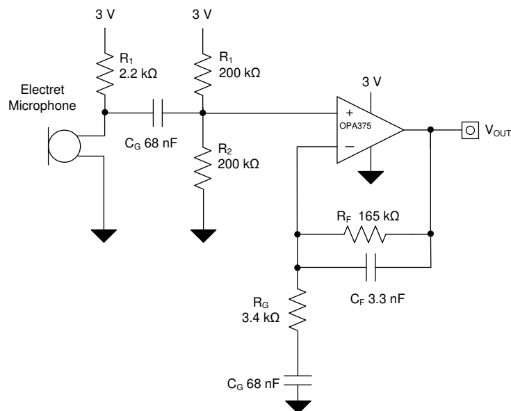
图 9-1. Microphone Preamplifier
