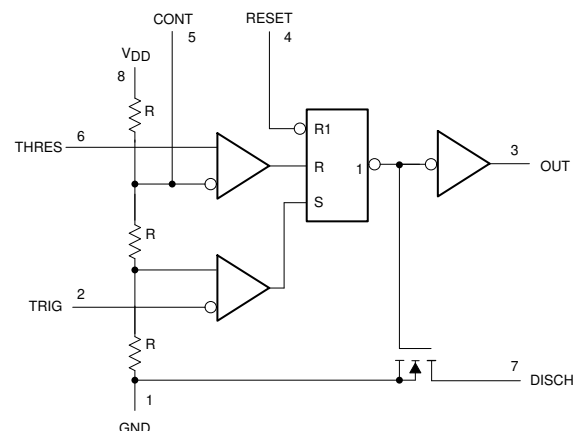
简化原理图
