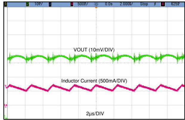
图 9-17. Output Ripple
