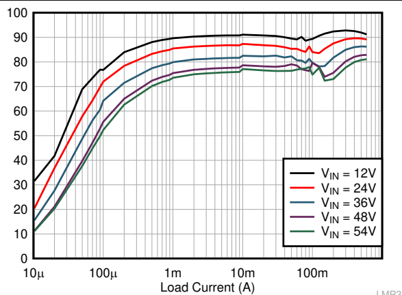
图 9-6. Efficiency
