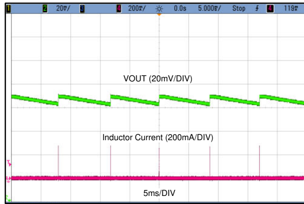
图 9-16. Output Ripple
