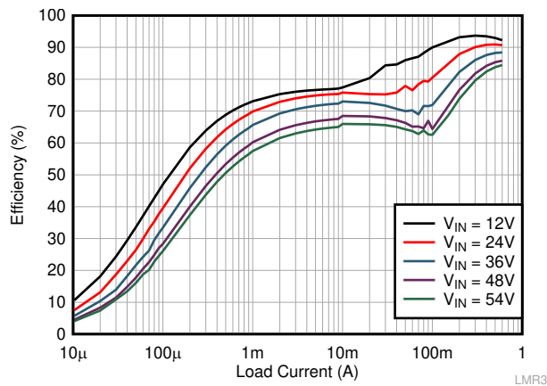
图 9-4. Efficiency
