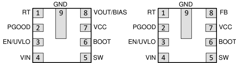
图 6-1. RPE Package 9-Pin (2 mm x 2 mm) VQFN-HR Top View
