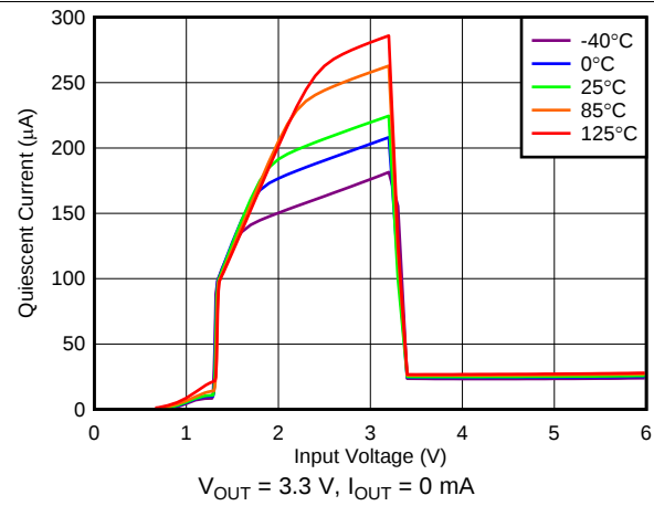
图 20. I_{GND} vs V_{IN}
