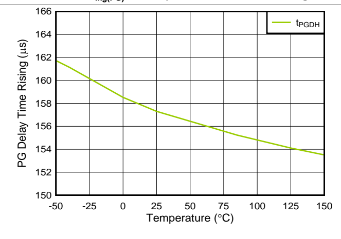
图 18. t_{PGDH} vs Temperature
