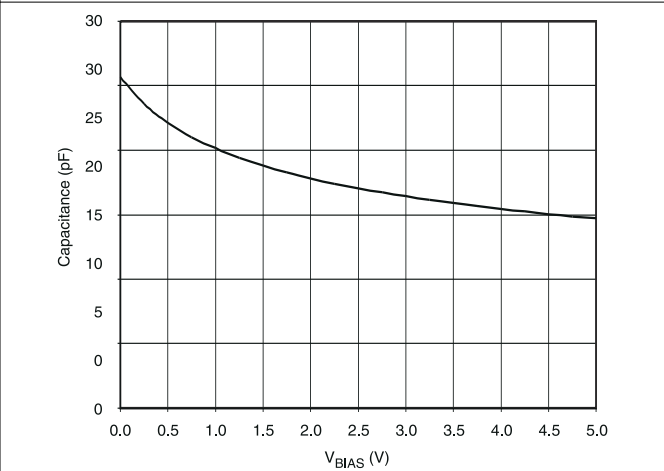
图 6-6. C1 or C2 Capacitance vs V_{BIAS}
