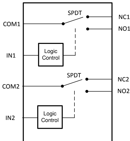
功能方框图
