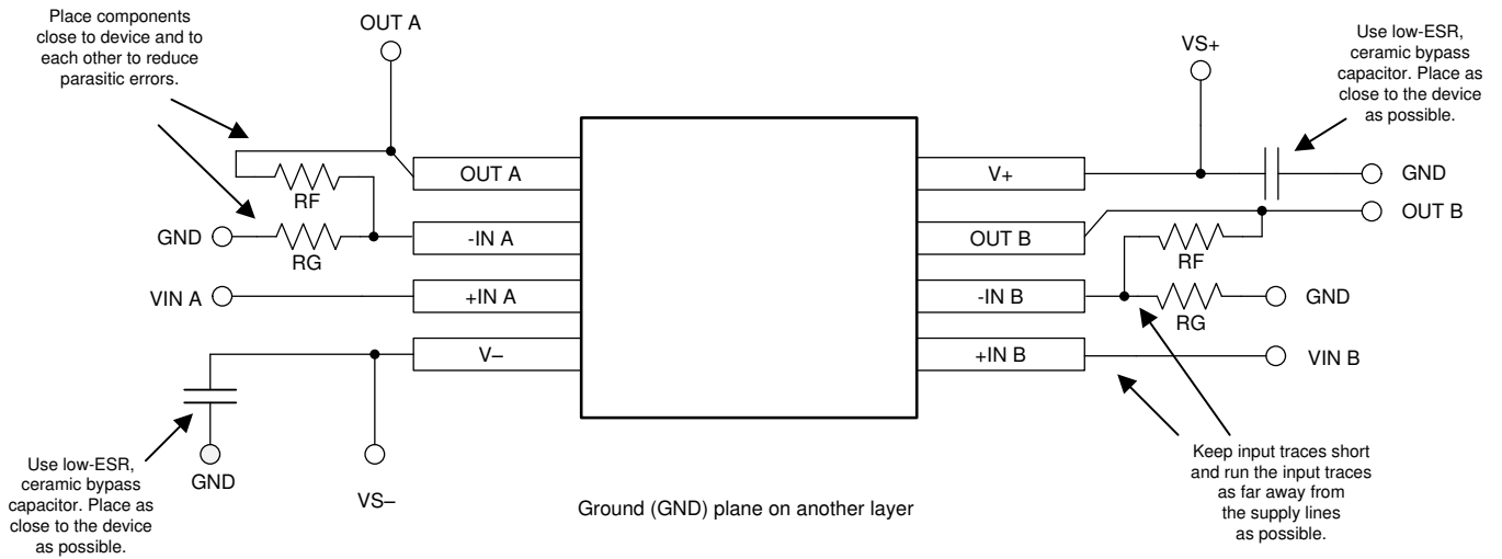
图 57. Layout Example
