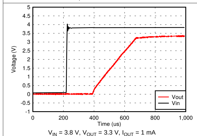
图 23. VIN Power-Up
