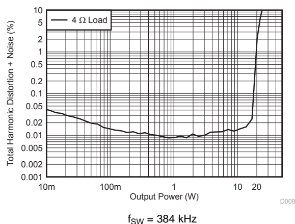
图 7. THD+N vs Power
