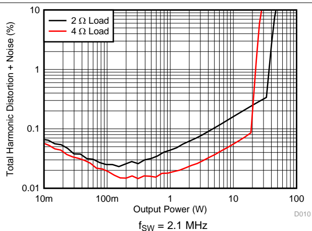
图 8. THD+N vs Power
