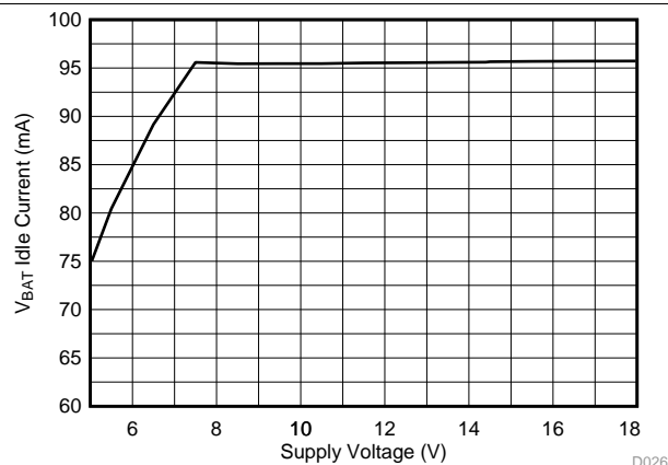
图 17. VBAT Idle Current vs Voltage
