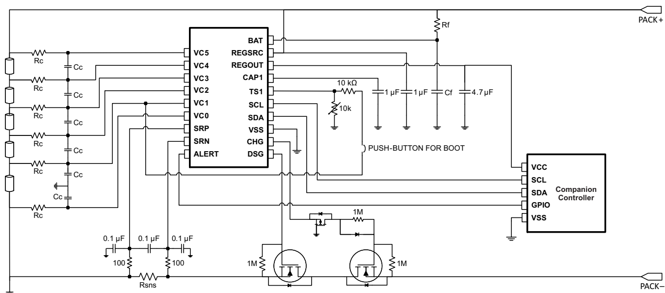
图 8-1. bq76920 与 bq78350 伴生控制器 IC
