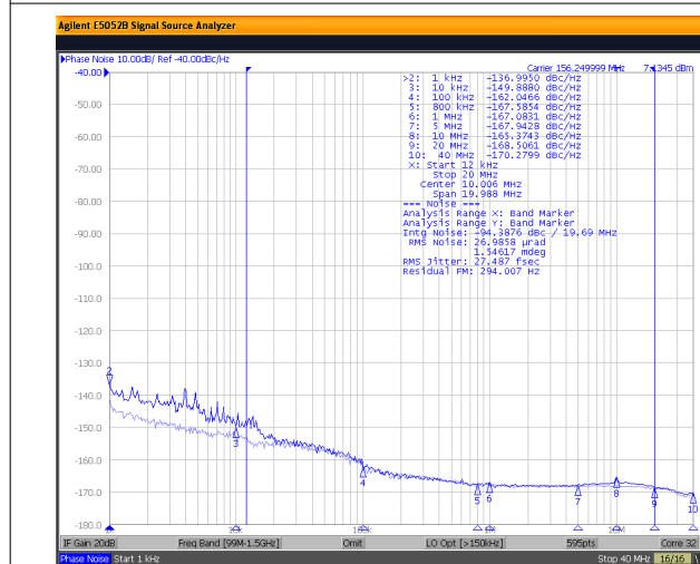
图 9-4. LMK1C110x 2.5-V Output Phase Noise 27.5-fs (12 kHz to 20 MHz)
