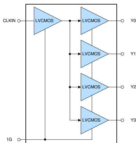
功能方框图
