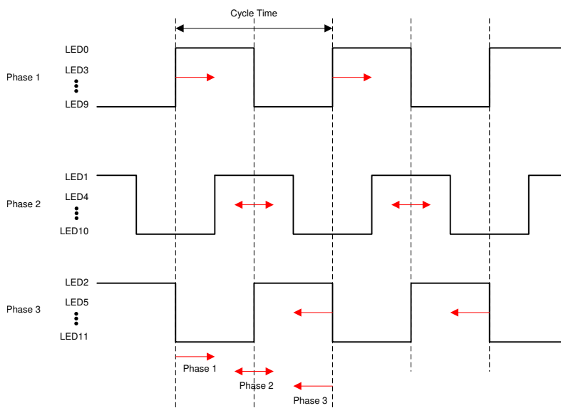
图 12. PWM Phase-Shifting
