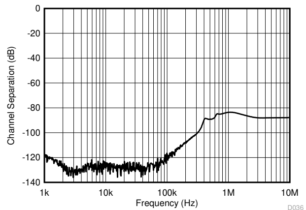
图 7-36. Channel Separation
