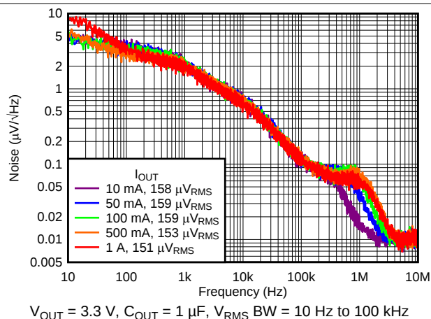
图 5. Output Spectral Noise Density
