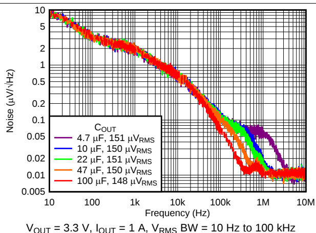
图 4. Output Spectral Noise Density
