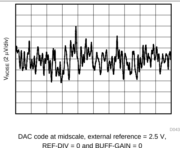
图 45. DAC Output Noise 0.1 Hz to 10 Hz
