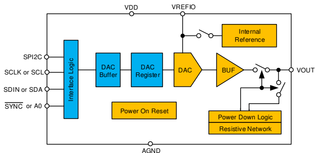
功能方框图
