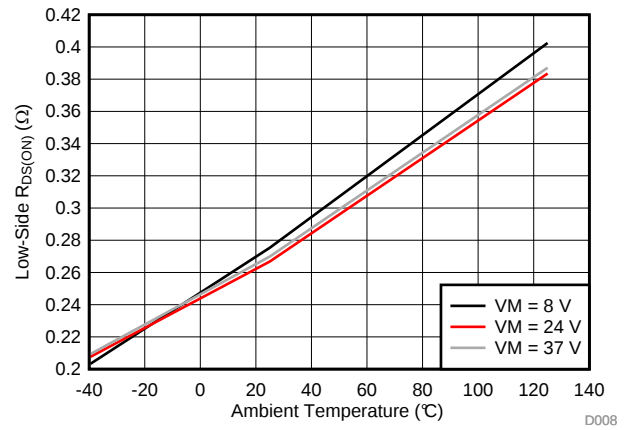
图 9. 低侧 R_{DS(ON)} 与温度间的关系
