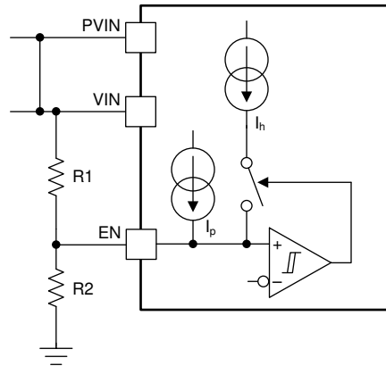
图 24. Adjustable V_{IN} and PV_{IN} UVLO
