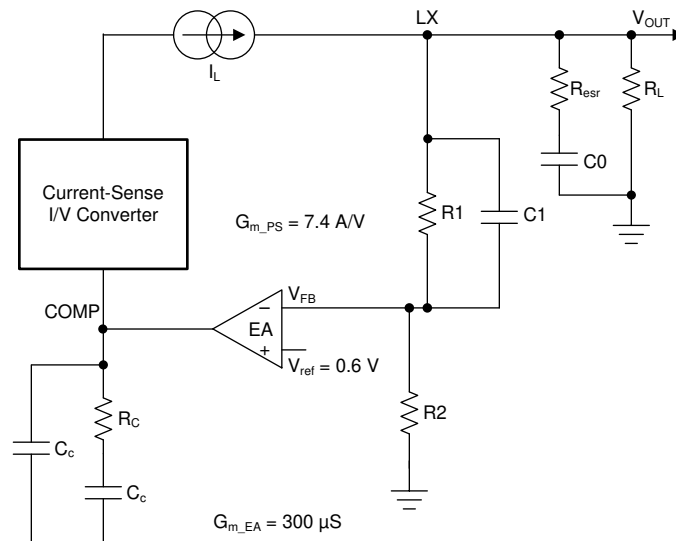
图 33. DC-DC Loop Compensation
