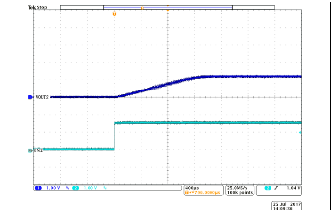
图 35. BUCK2 Soft-Start
