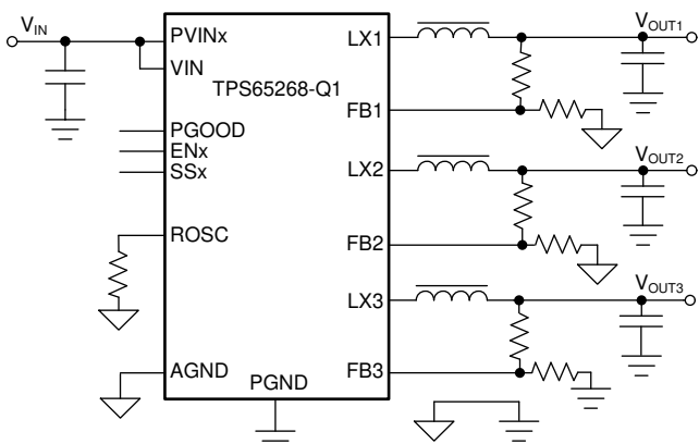
应用原理图
