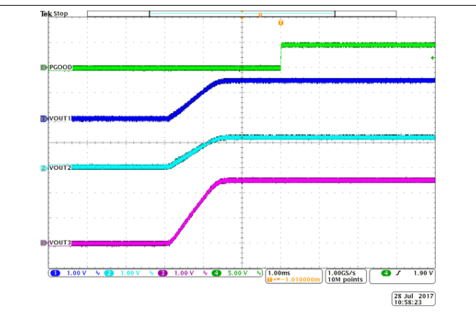
图 49. PGOOD
