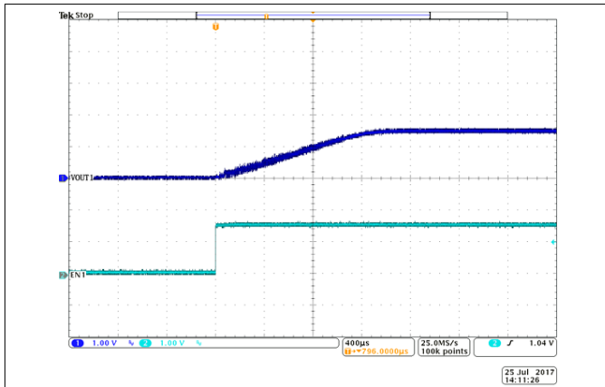
图 34. BUCK1 Soft-Start
