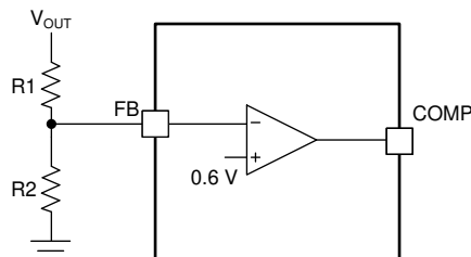
图 21. Voltage Divider Circuit
