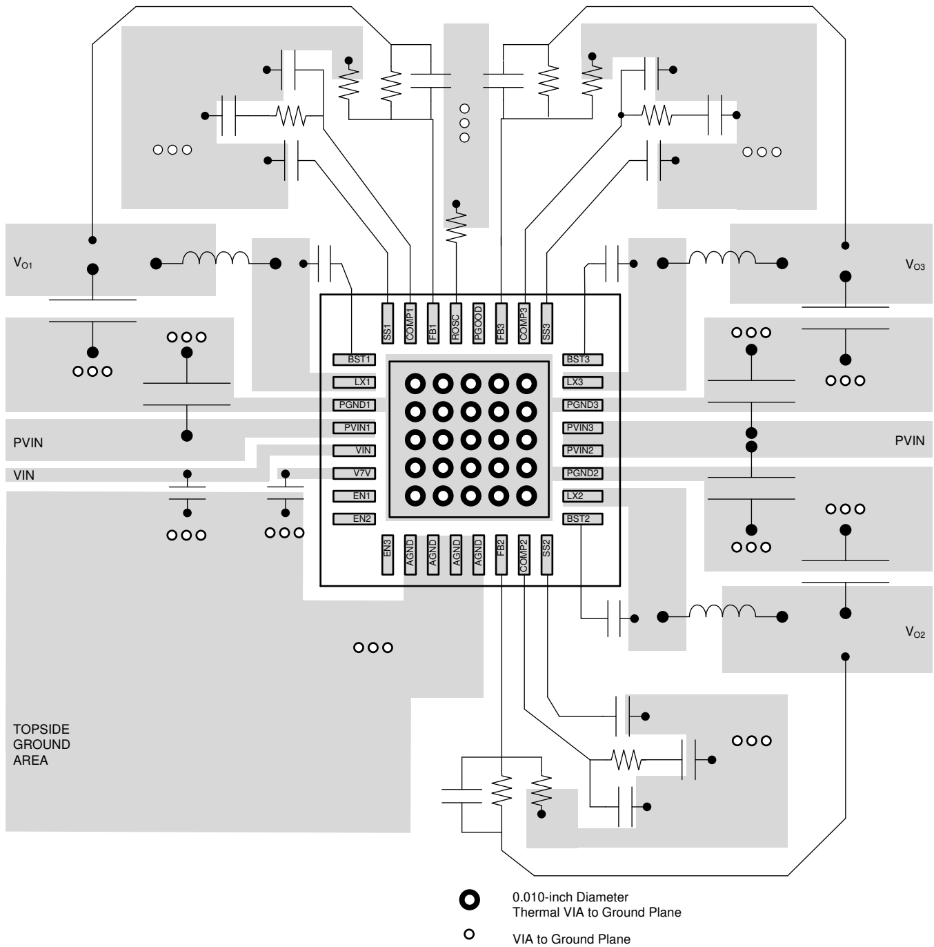
图 53. PCB Layout
