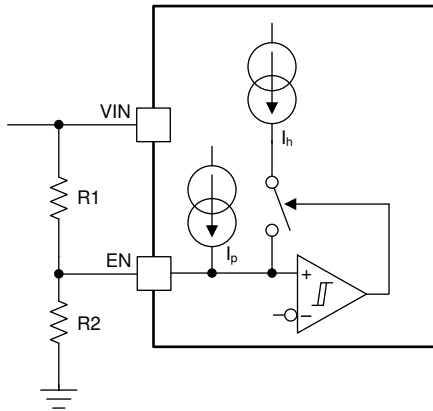
图 22. Adjustable V_{IN} UVLO
