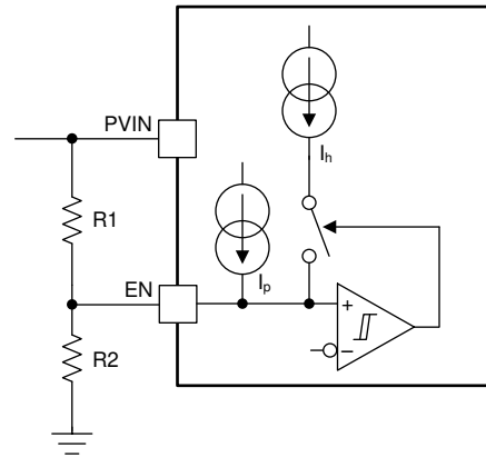
图 23. Adjustable PV_{IN} UVLO, V_{IN} > 4 V
