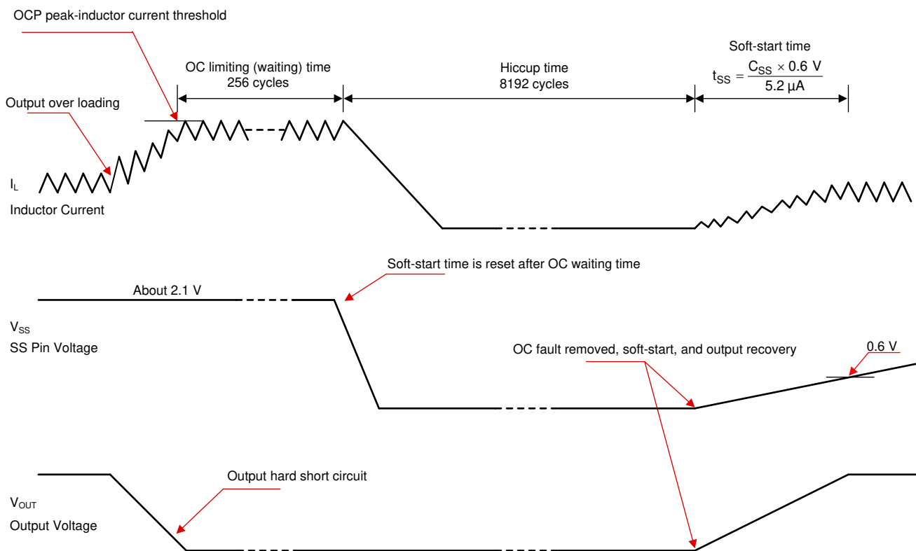
图 29. Overcurrent Protection
