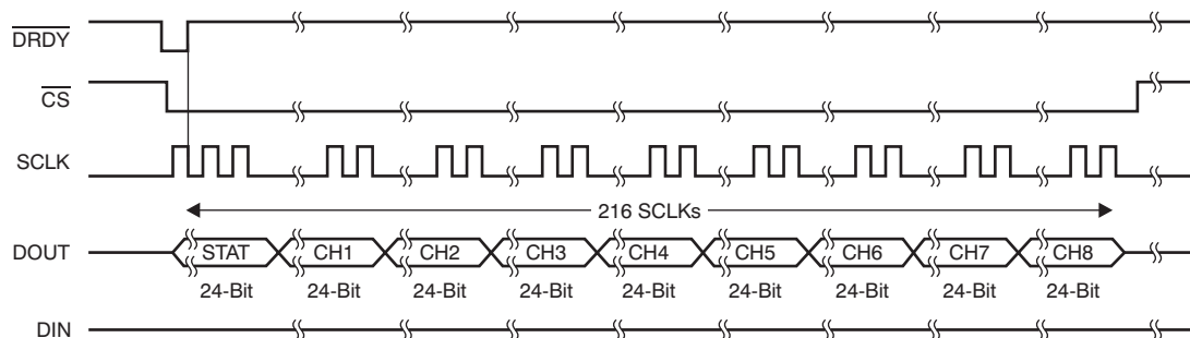
Figure 69. ADS1298 的 SPI 总线数据输出 (八个通道)
