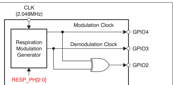
Figure 48. 外部呼吸 (RESP_CTRL = 01b) 方框图
