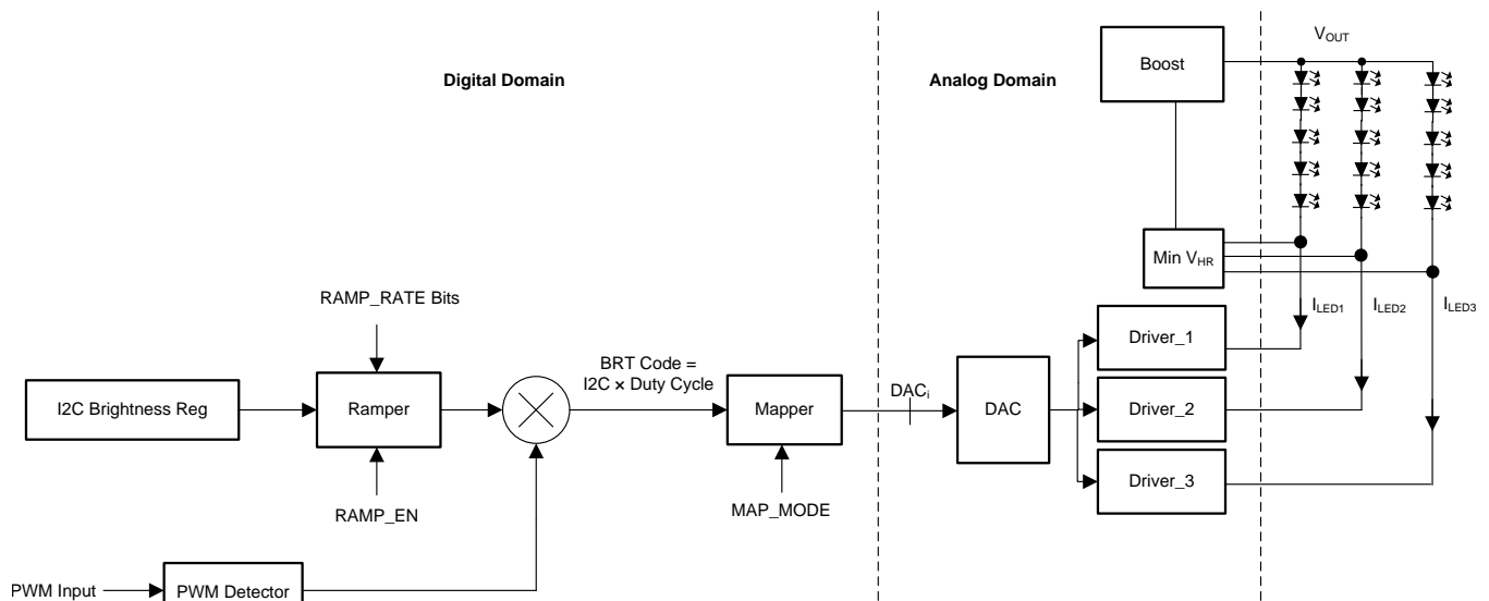
图 27. Brightness Control 11 (I 2 C + PWM)
