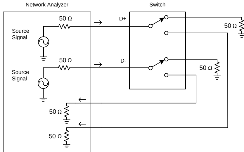
图 10. Off Isolation
