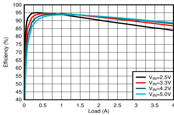
图 9-11. Efficiency
