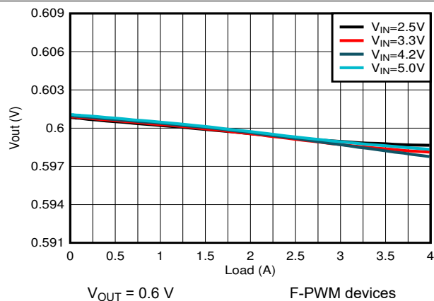
图 9-6. Load Regulation
