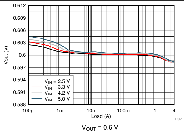
图 9-4. Load Regulation
