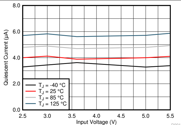
图 7-4. Quiescent Current
