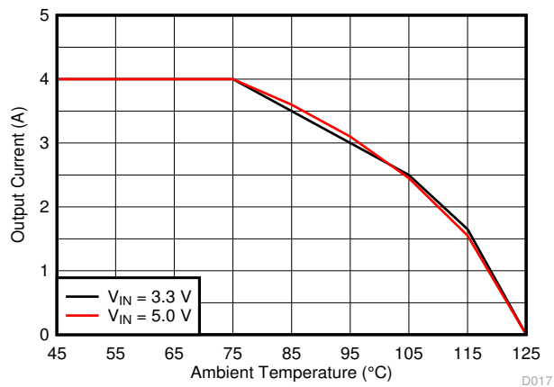
图 9-29. Thermal Derating
