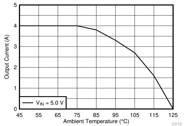
图 9-30. Thermal Derating
