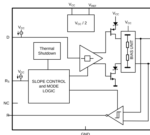
等效输入和输出原理图
