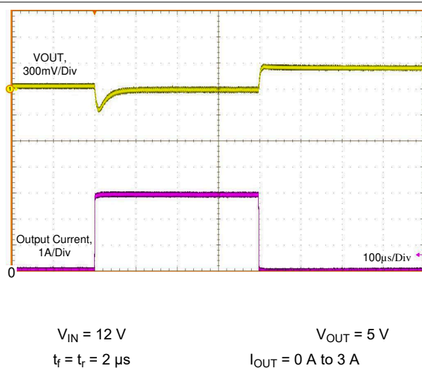
图 8-15. Load Transient
