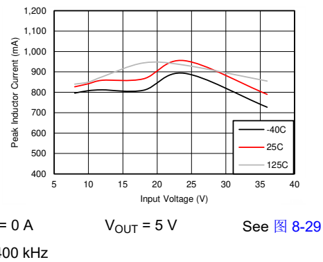
图 6-6. I_{PEAK-MIN}
