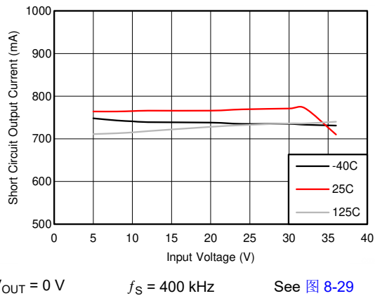
图 6-3. Short-Circuit Output Current
