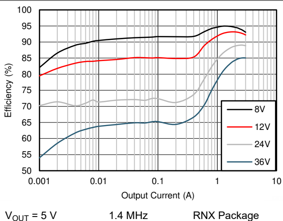
图 8-7. Efficiency
