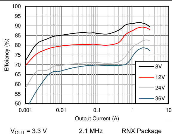
图 8-10. Efficiency
