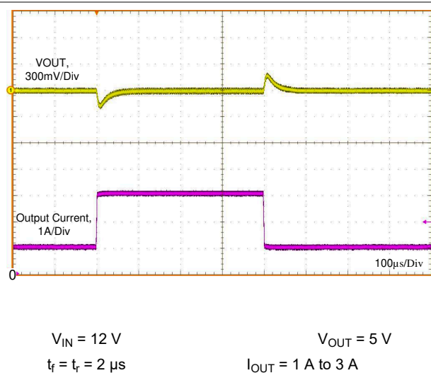
图 8-16. Load Transient
