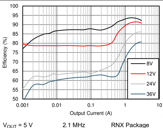
图 8-9. Efficiency
