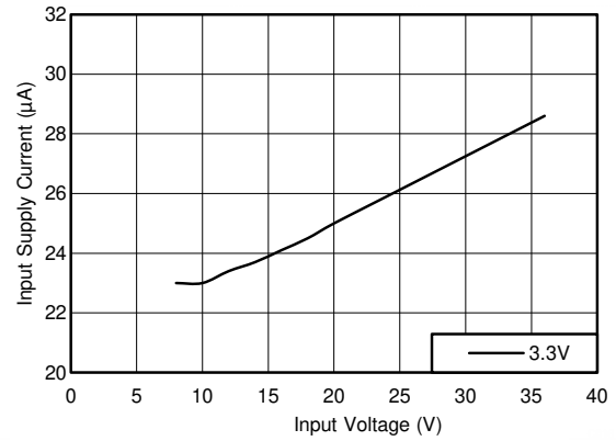
图 8-18. Input Supply Current
