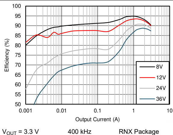
图 8-6. Efficiency
