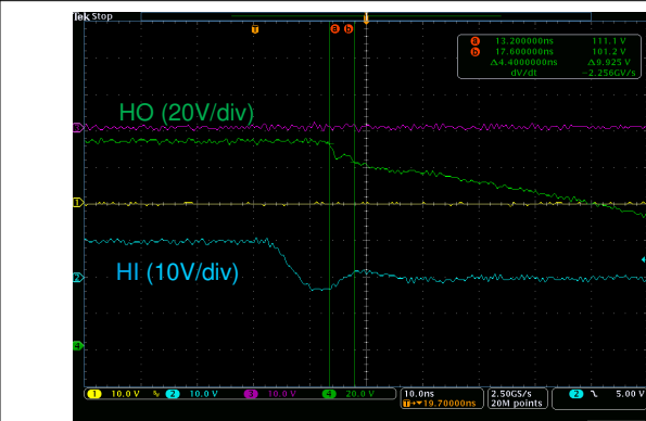
V DD =12 V, HS=100V
