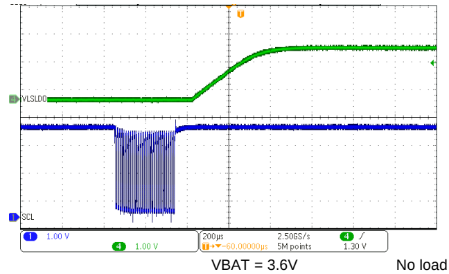
图 95. LDO Enable Through I²C (EN_LS_LDO)
