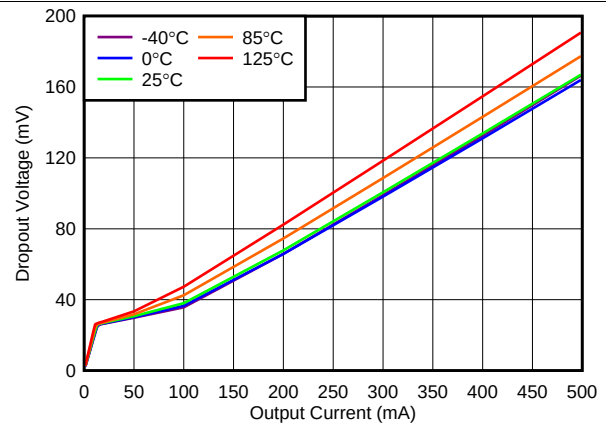
图 14. 5.0-V Dropout Voltage vs I_{OUT}
