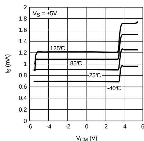
图 30. I_{\text{S}} 与 V_{\text{CM}} 间的关系 (LM7321)
