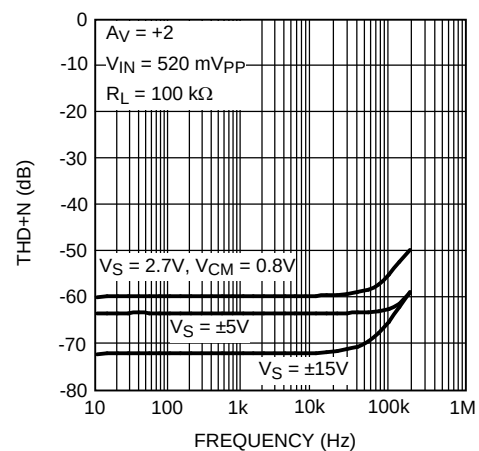
图 54. THD+N 与频率间的关系
