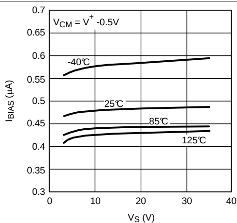
图 27. I_{\text{BIAS}} 与 V_{\text{S}} 间的关系
