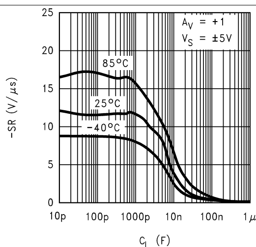
图 63. -SR 与容性负载间的关系
