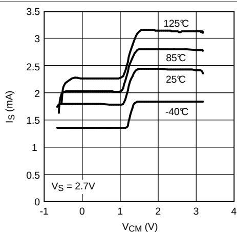
图 29. I_{\text{S}} 与 V_{\text{CM}} 间的关系 (LM7322)
