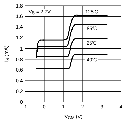
图 28. I_{\text{S}} 与 V_{\text{CM}} 间的关系 (LM7321)
