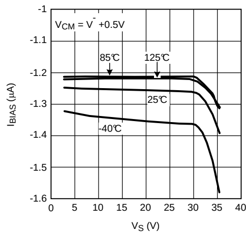
图 26. I_{\text{BIAS}} 与 V_{\text{S}} 间的关系
