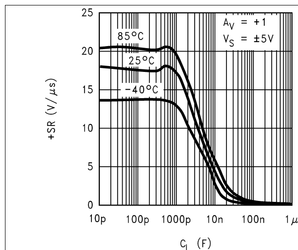
图 62. +SR 与容性负载间的关系
