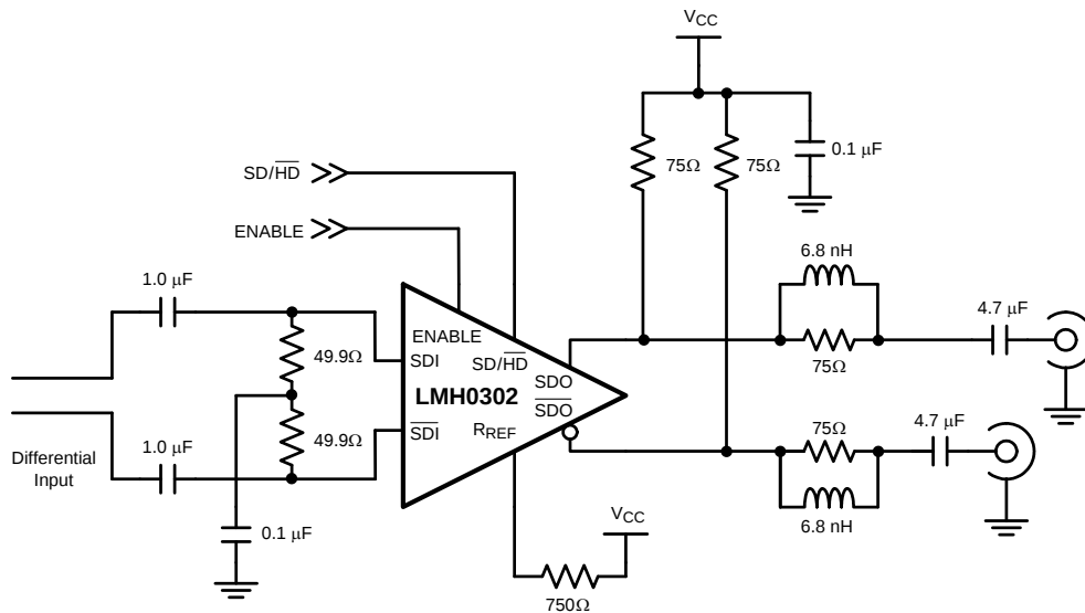
典型应用
