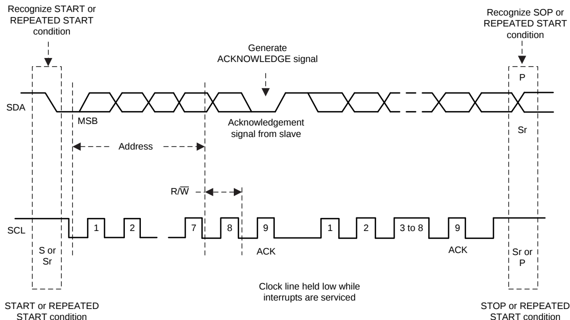
图 5-20. Bus Protocol
