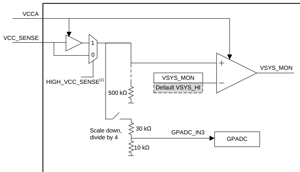
图 5-27. VSYS_MON Comparator Details
