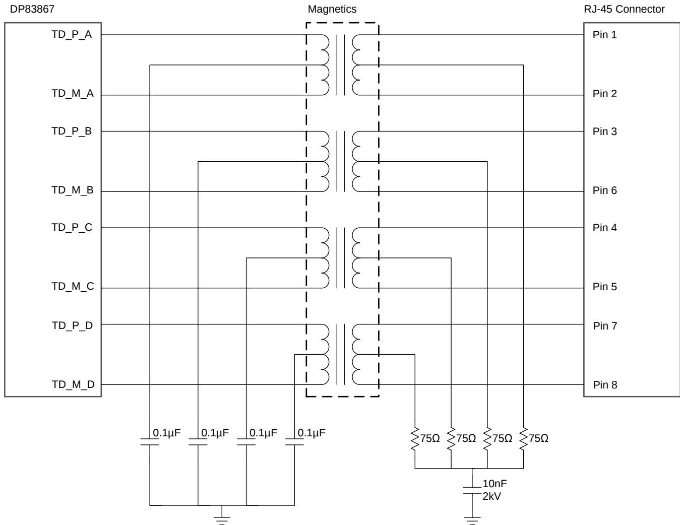
图 26. Magnetics Connections
