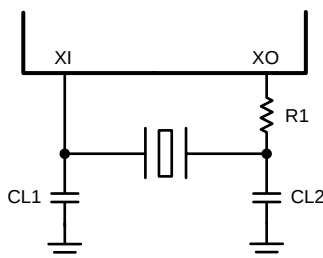
图 28. Crystal Oscillator Circuit
