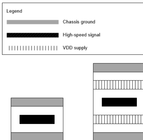
图 35. Alternative Layer Stack Up
