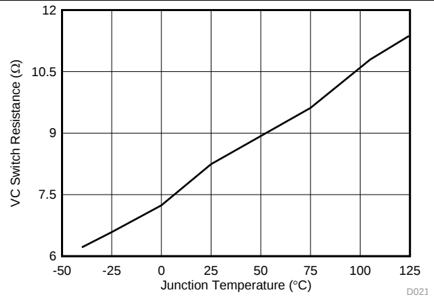
Figure 20. VC 开关电阻与温度间的关系
