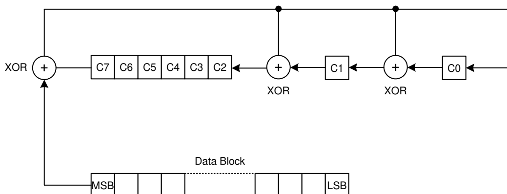
图 8-19. CRC Module
