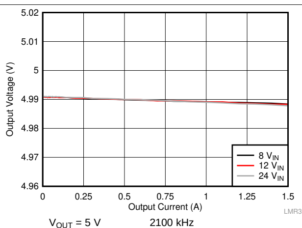
图 47. Load Regulation
