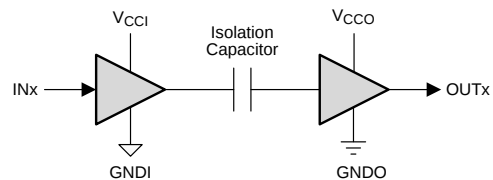
简化原理图
