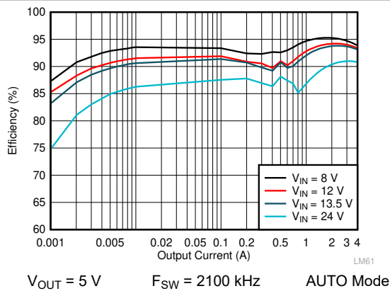
图 10-7. LM61440-Q1 Efficiency
