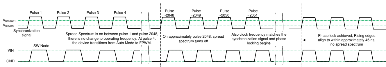
图 9-4. Synchronization Process
