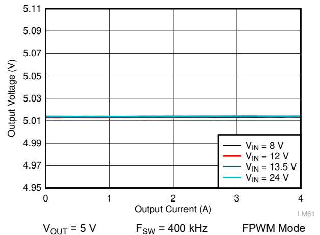
图 10-14. LM61440-Q1 Load and Line Regulation
