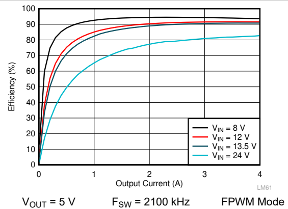
图 10-8. LM61440-Q1 Efficiency
