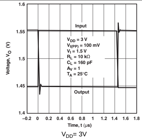
图 46. 反相小信号
